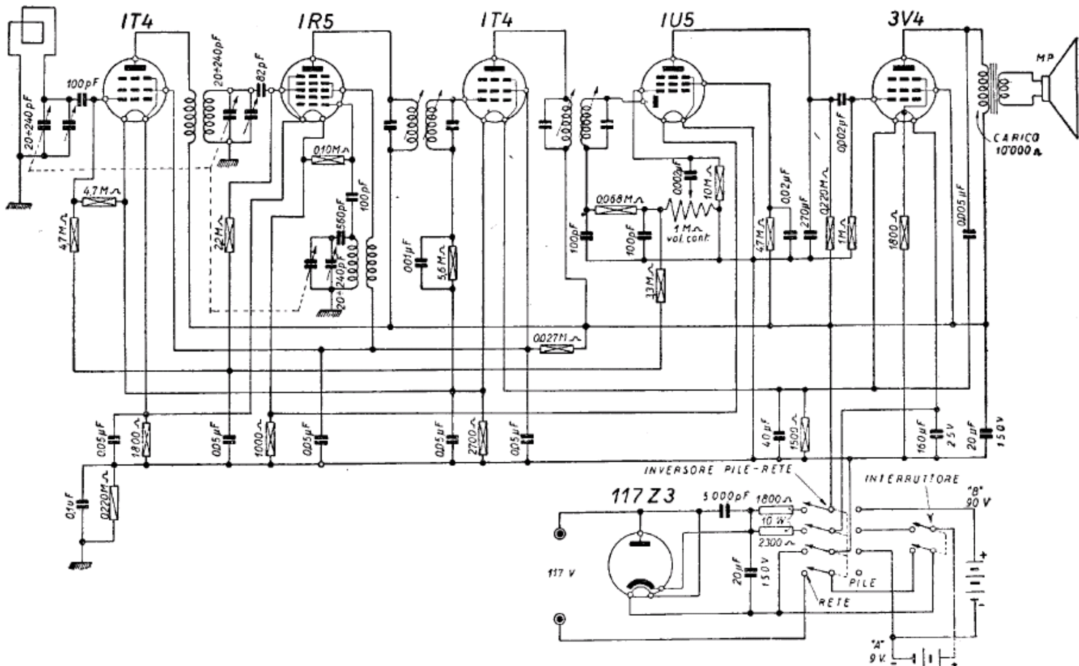
- Schema di portatile "tre correnti", alimentabile con pile o rete-luce CA/CC.
